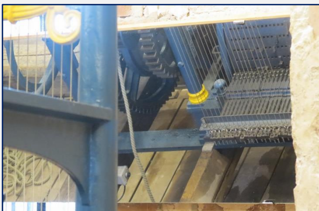
Detail speeltrommel met bedieningslijnen
